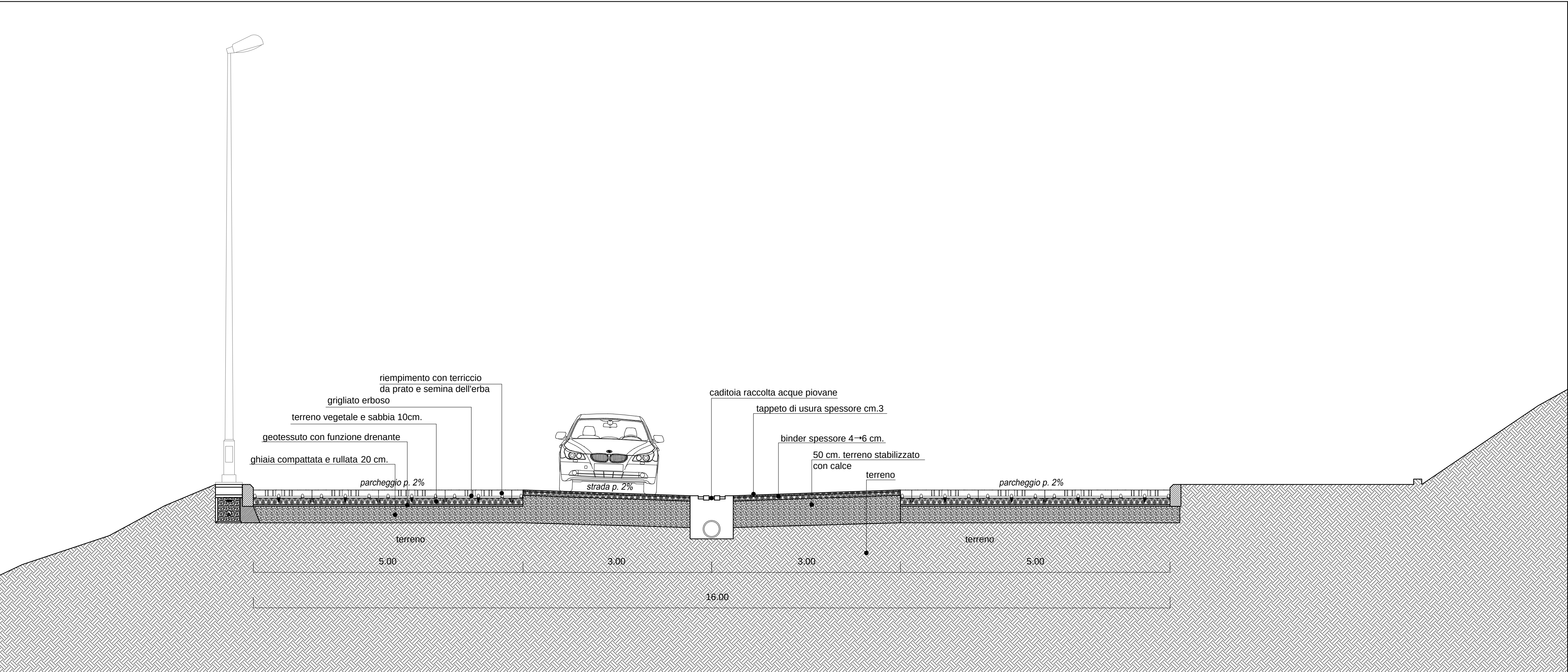
SEZIONE A-A PARCHEGGIO PUBBLICO scala 1:50
