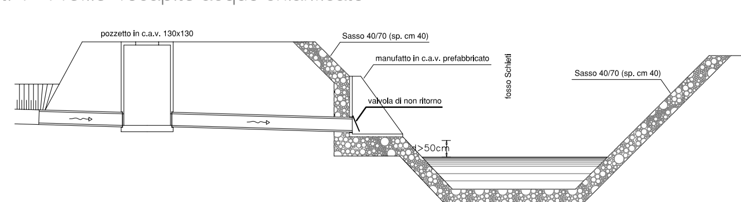
det. 1 - Profilo -recapito acque chiarificate
