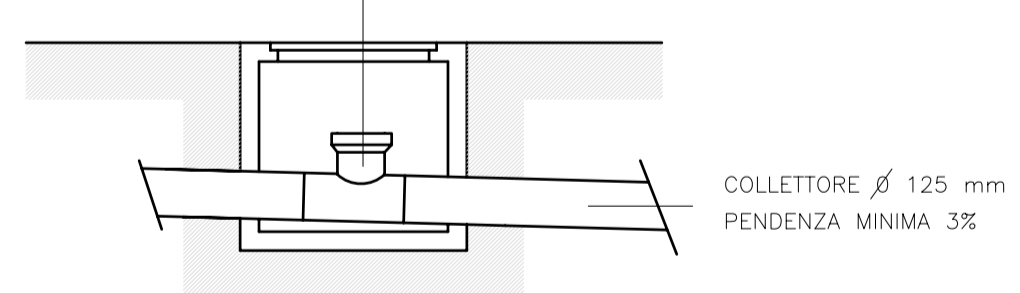
det. 1 - pianta- Recapito acque chiarificate
