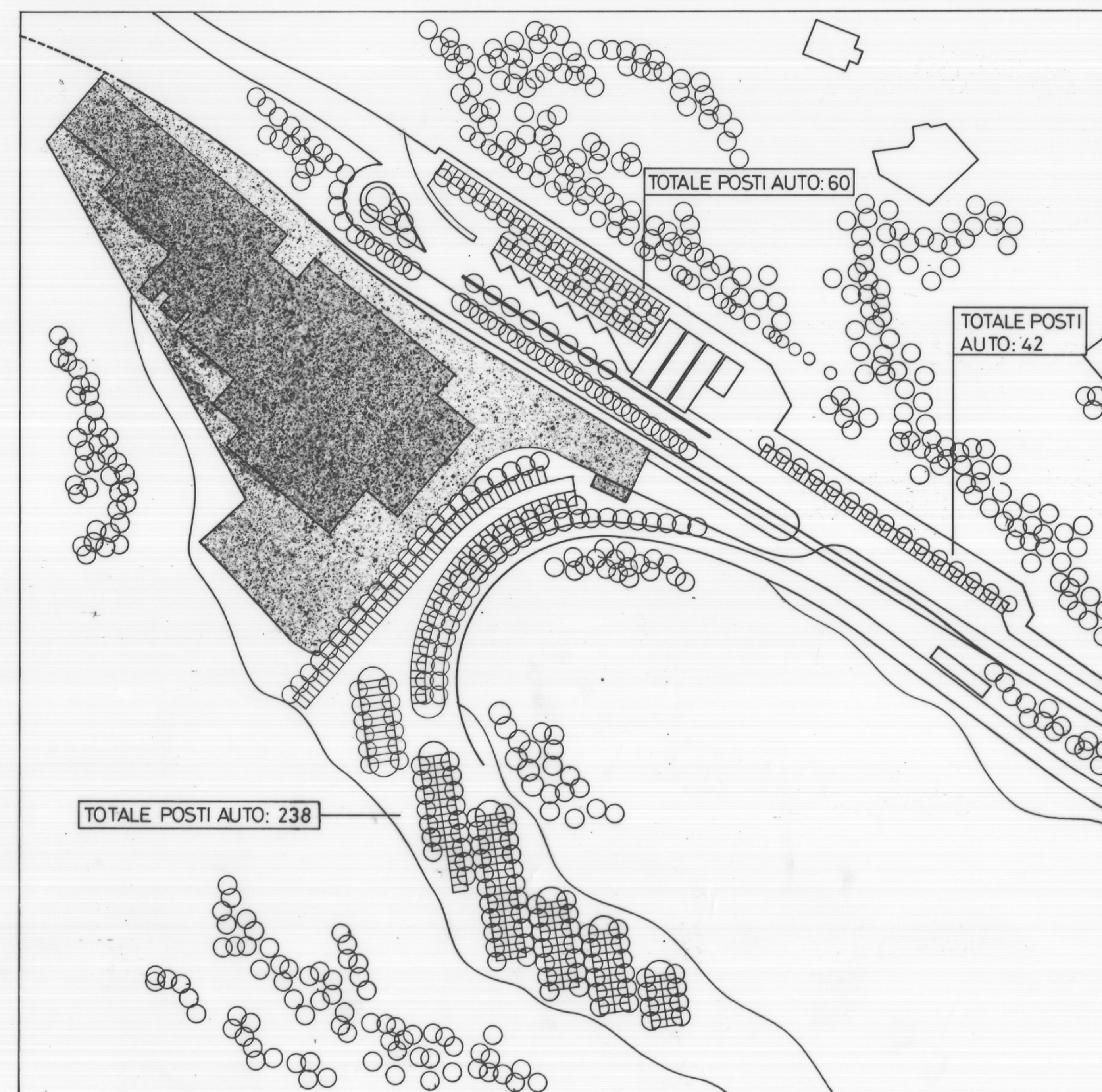
FASE 1: STAZIONE AUTOCORRIERE E TRENO
