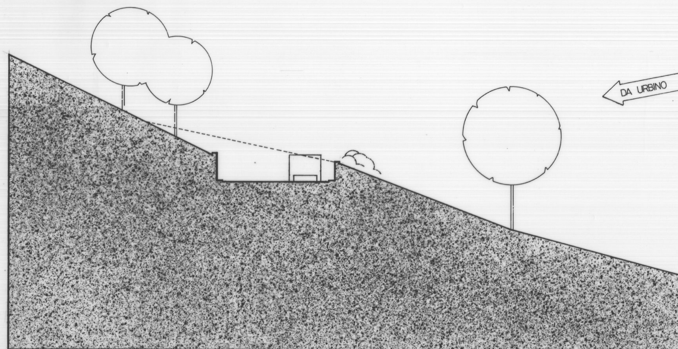
NUOVO TRATTO STRADALE: IPOTESI DI SEZIONE
