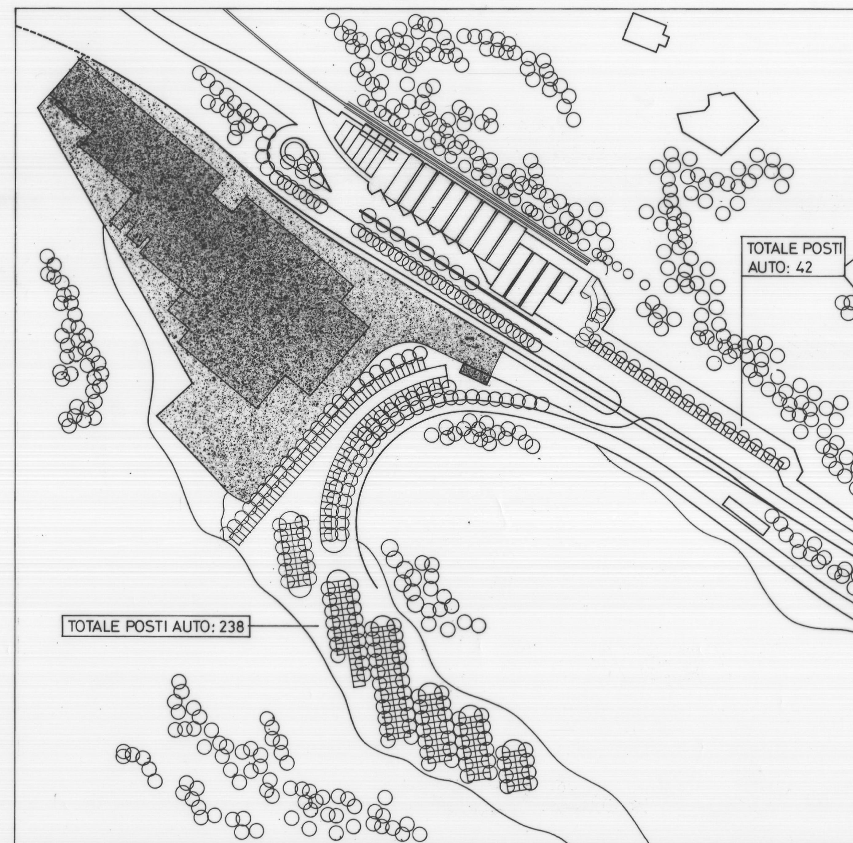
FASE 3: STAZIONE, GRANDE MAGAZZINO E LABORATORI ARTIGIANI
